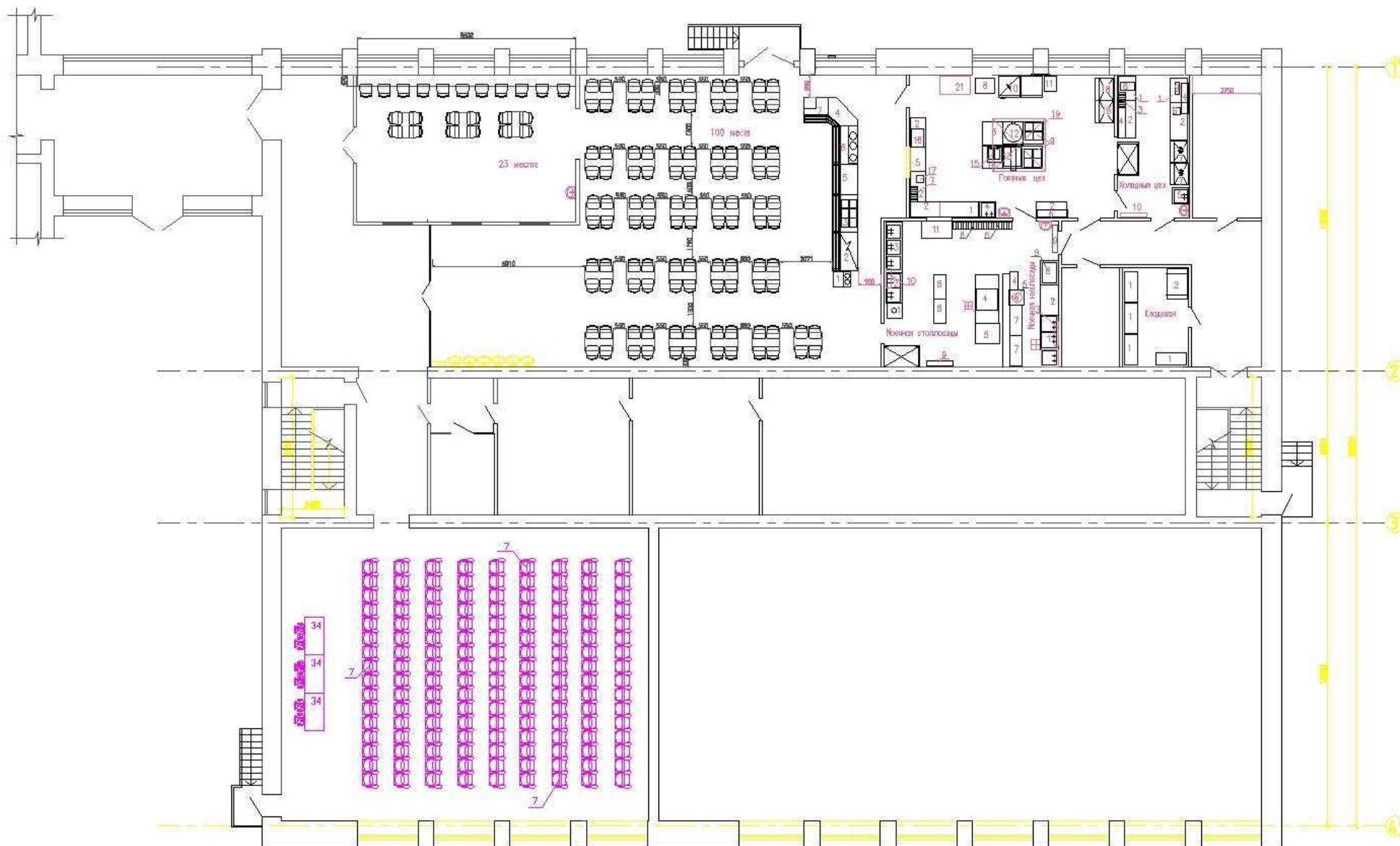
План 1-го этажа (Литер А1,а19) на отм. +3.500 М 1:100
